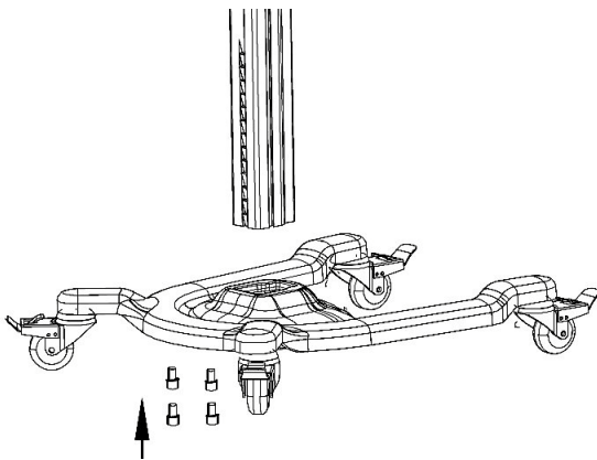
Abb. 5: Montage der Säule am Fahrgestell
