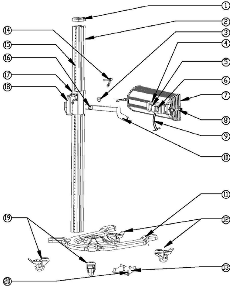
Abb. 9: Ersatzteilzeichnung 7550 IR-1
