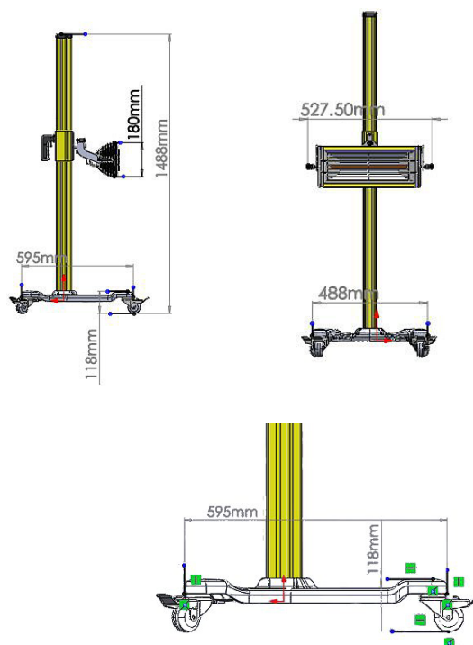
Abb. 4: Maße für den Einsatzbereich
