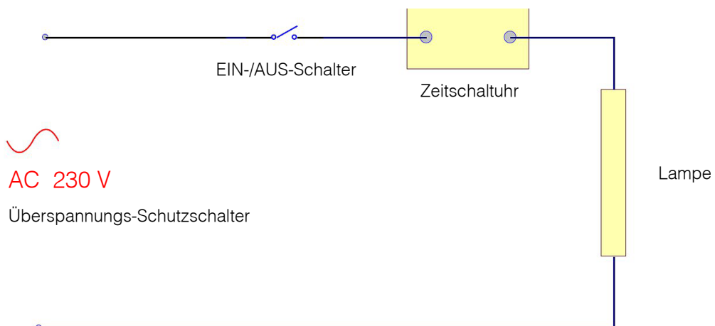
Abb. 10: Elektro-Schaltplan
