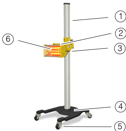
Abb. 3: Infrarot-Lackrockner 7550 IR-1
